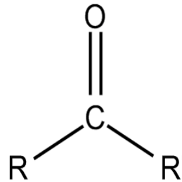
KETONE
